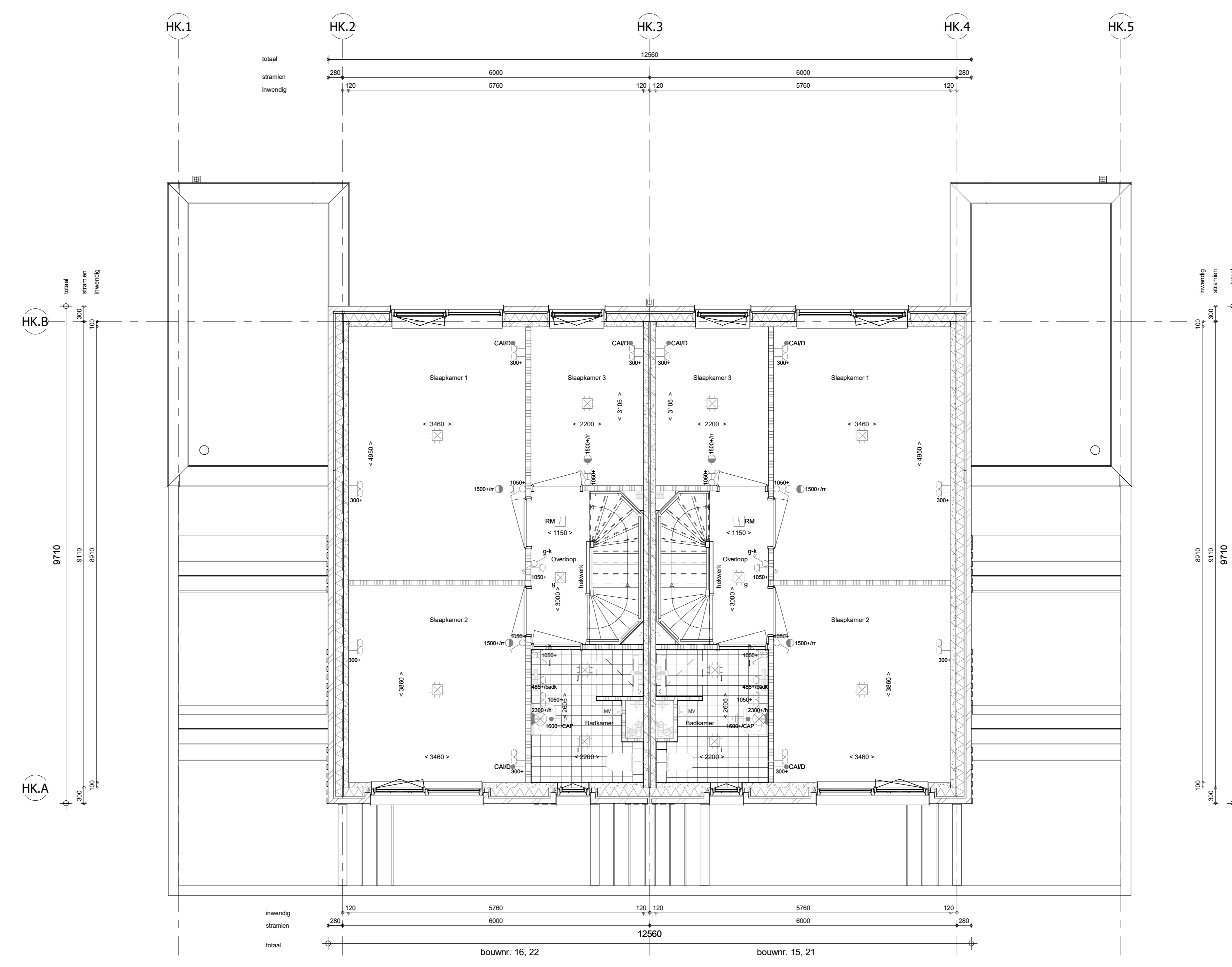
1e verdieping 1:50
