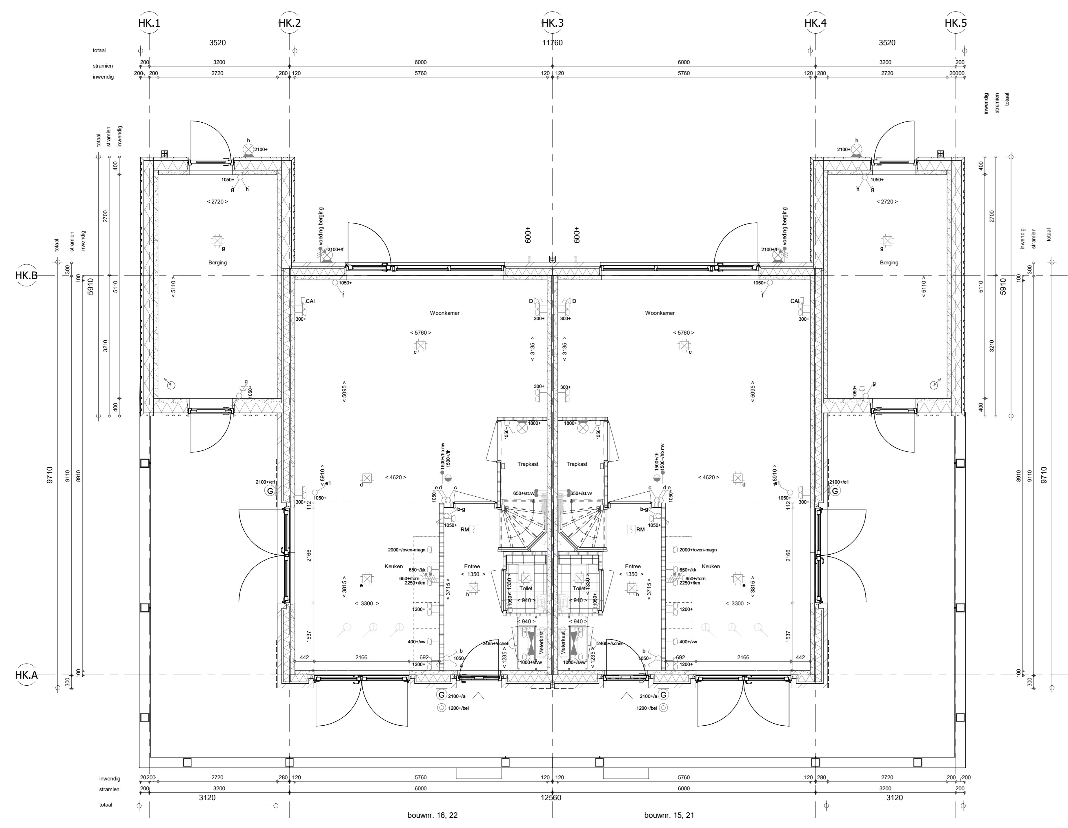
begane grond 1:50
